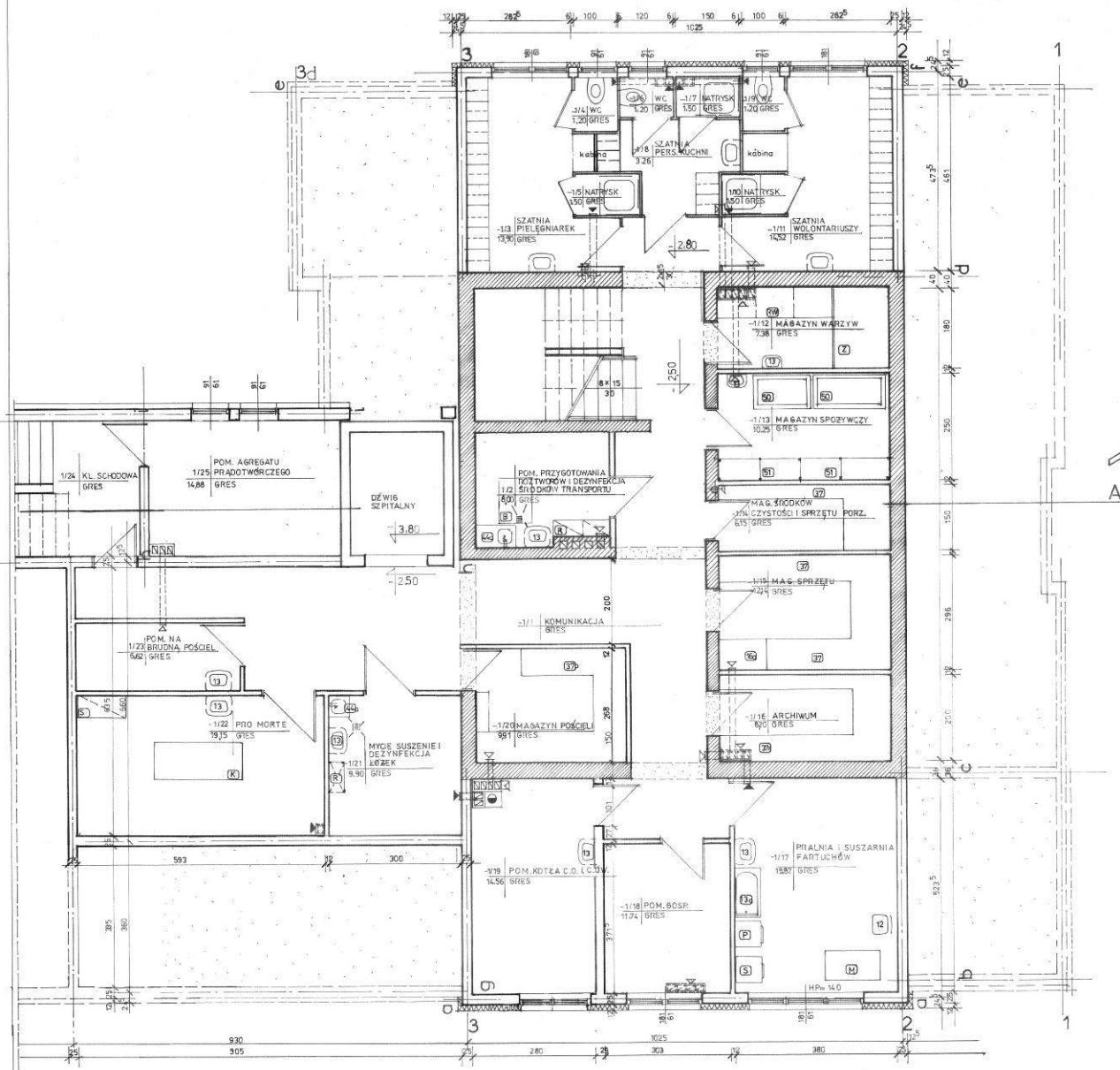
RZUT PIWNIC 1:50
